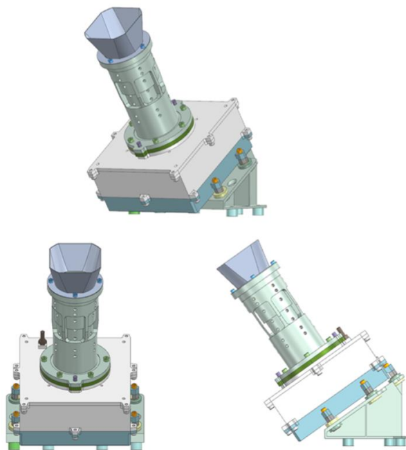
圖二：嫦娥七號月球著陸器寬視場望遠鏡相機ILO-C的詳細效果圖。
